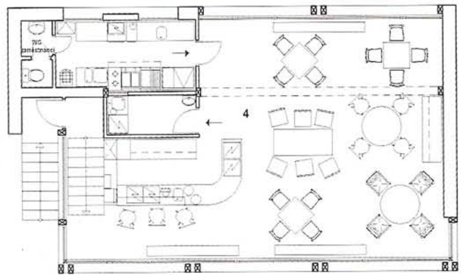
půdorys 2. NP
